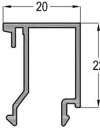
11-020 0,276 kg/mt
