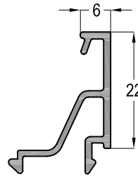
11-006 0,218 kg/mt
