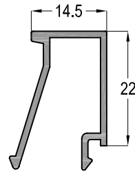
11-015 0,241 kg/mt
